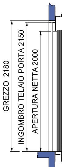
SEZIONE TELAI PORTE NF (EI120)
