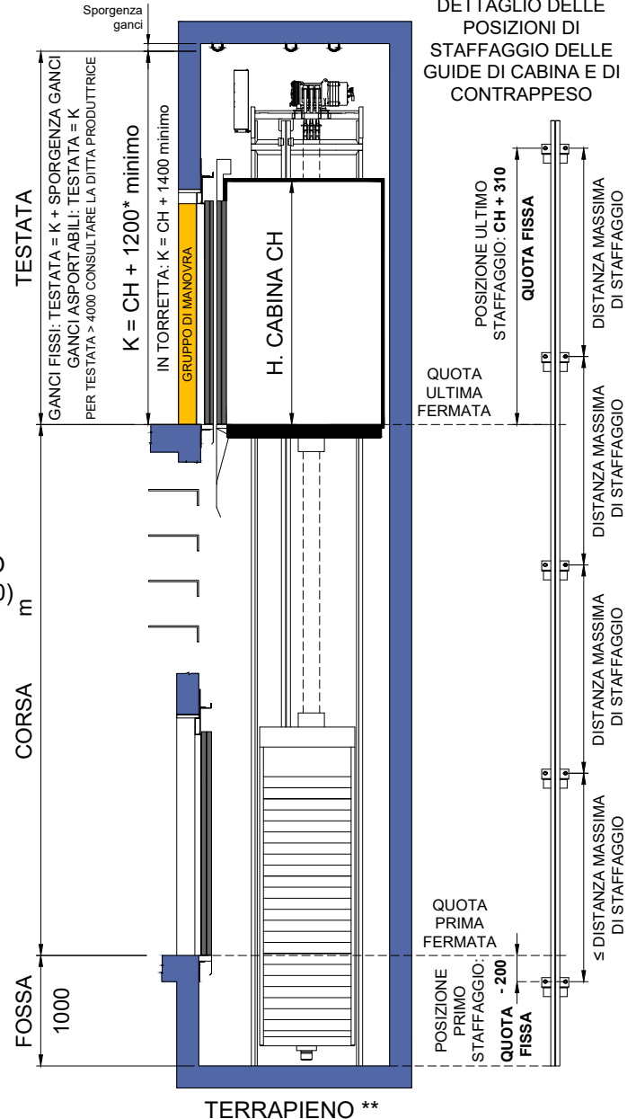
SEZIONE VANO CORSA
