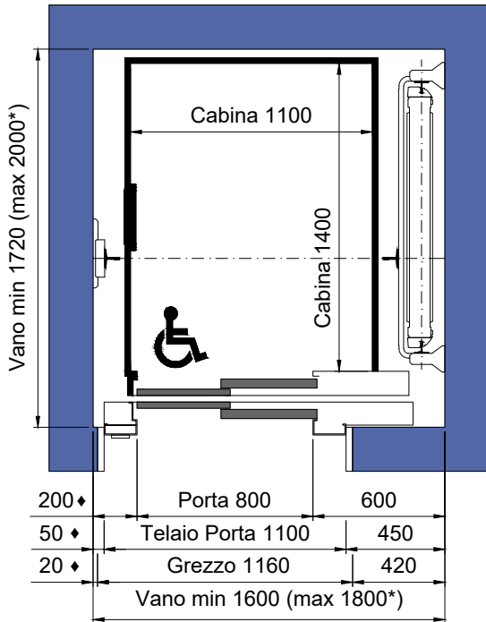
PIANTA VANO CORSA TELAIO PORTE MRF 150
