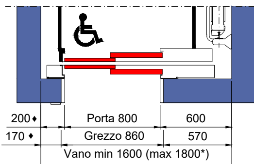
PIANTA VANO CORSA TELAIO PORTE NF (EI120)
