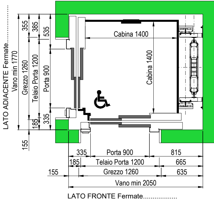
PIANTA VANO CORSA TELAIO PORTE DA 150mm
