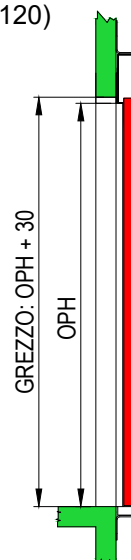
SEZIONE PORTE SENZA TELAIO (E1120)
