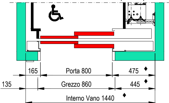
PIANTA VANO CORSA PORTE SENZA TELAIO (E120)
